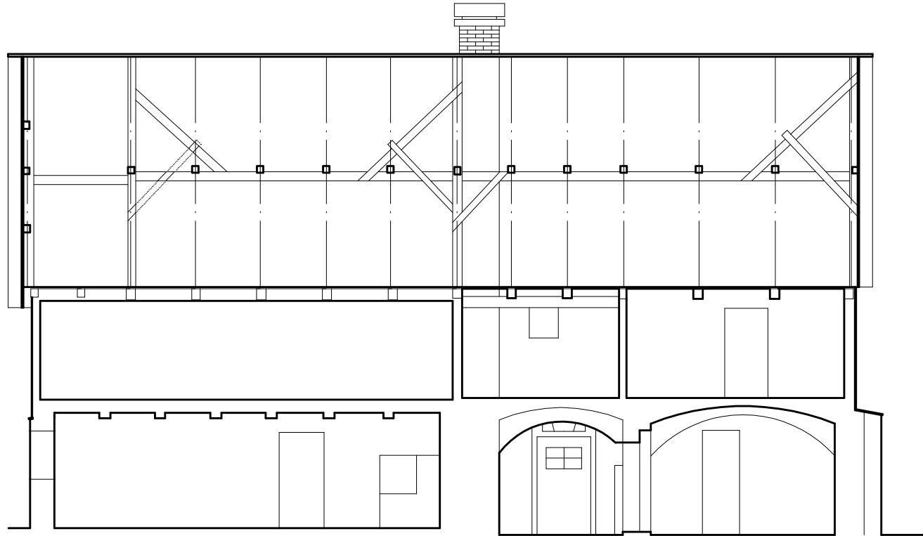
PODÉLNÝ ŘEZ A-Á
